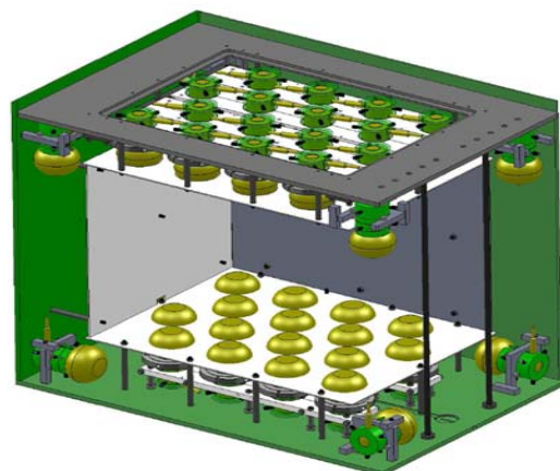
Desenho Final do Detector do Projeto Neutrinos Angra
